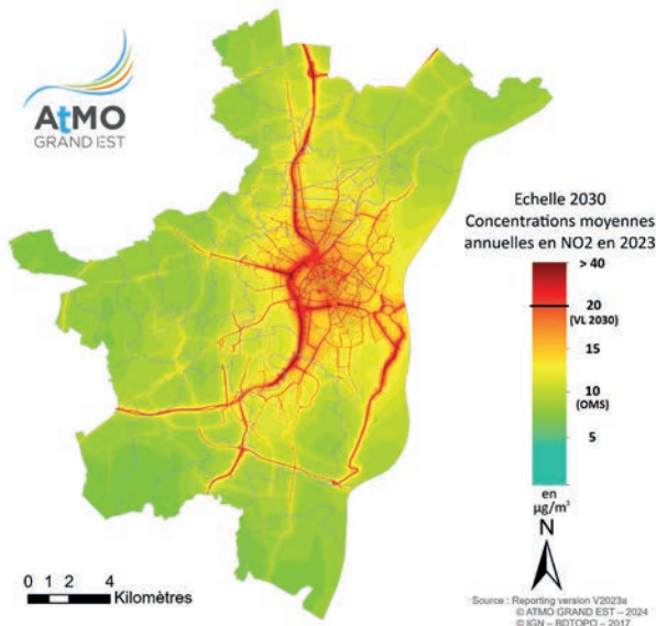
CONCENTRATION MOYENNE ANNUELLE DE NO2 - SEUIL PROJETÉ 2030 DE 20 µg/m³
