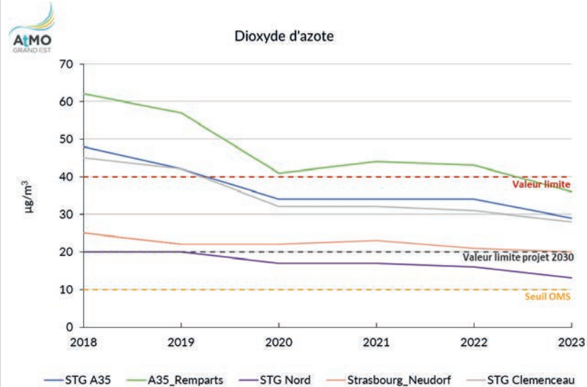
ÉVOLUTION DES CONCENTRATIONS EN DIOXYDE D'AZOTE DES STATIONS DE MESURE DE L'EUROMÉTROPOLE DE STRASBOURG - Source : ATMO Grand Est, 2024
