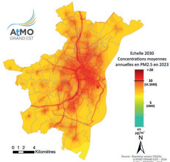
CONCENTRATION MOYENNE ANNUELLE DE PM 2.5 SEUIL PROJETÉ 2030 DE 10 µg/m³
